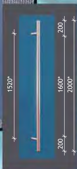
ART. 48.2000.V MAT. INOX \varnothing 48,3 x 1,6
