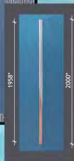
ART. 48.2000.H MAT. INOX \varnothing 48,3 x 1,6
