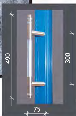
ART. 28.300.11.R.PK MAT. INOX \varnothing 28
